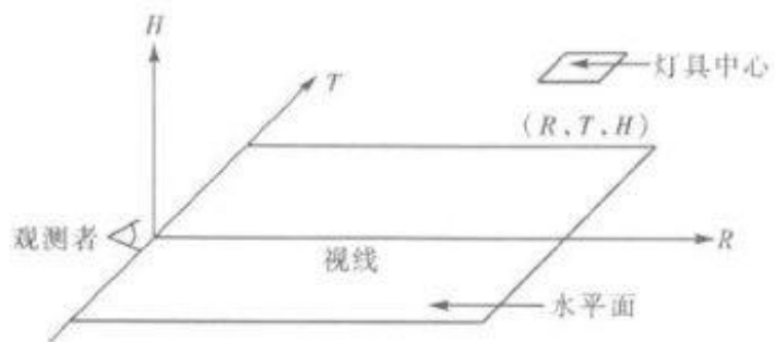
图 A.0.1 以观察者位置为原点的位置指数坐标系 (R, T, H) ，对灯具中心生成 H/R 和 T/R 的比值
