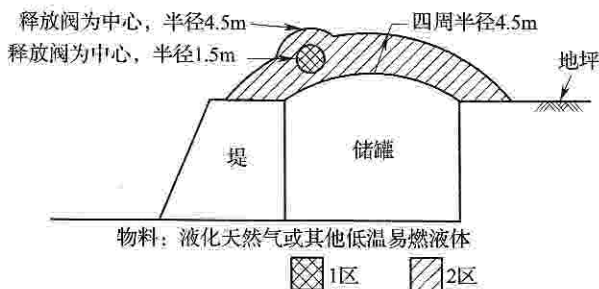
图 B. 0. 1-21 低温液化气体储罐
